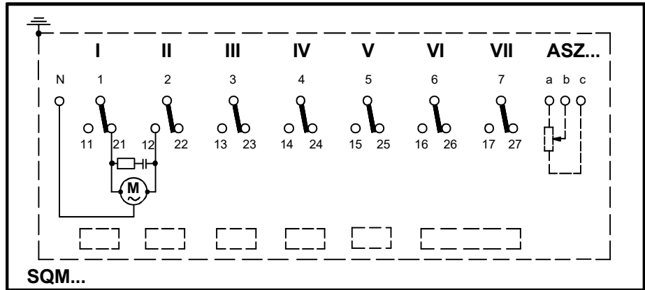
Схема № 1 (H 4 318 1521 0)
