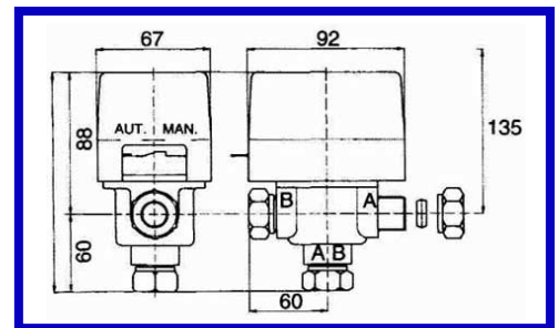
Ввод для Cu-трубок - B
